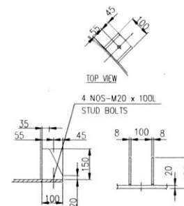
SUPPORT LEG DETAIL 45°, 135°, 225° & 315° SCALE : N.T.S.
