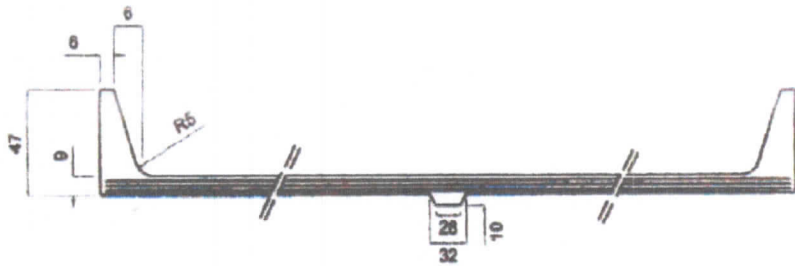
A - A
