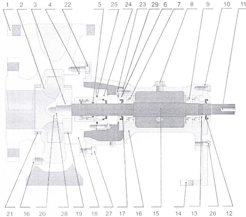
Pump Part List RZ SES SS316 Material
