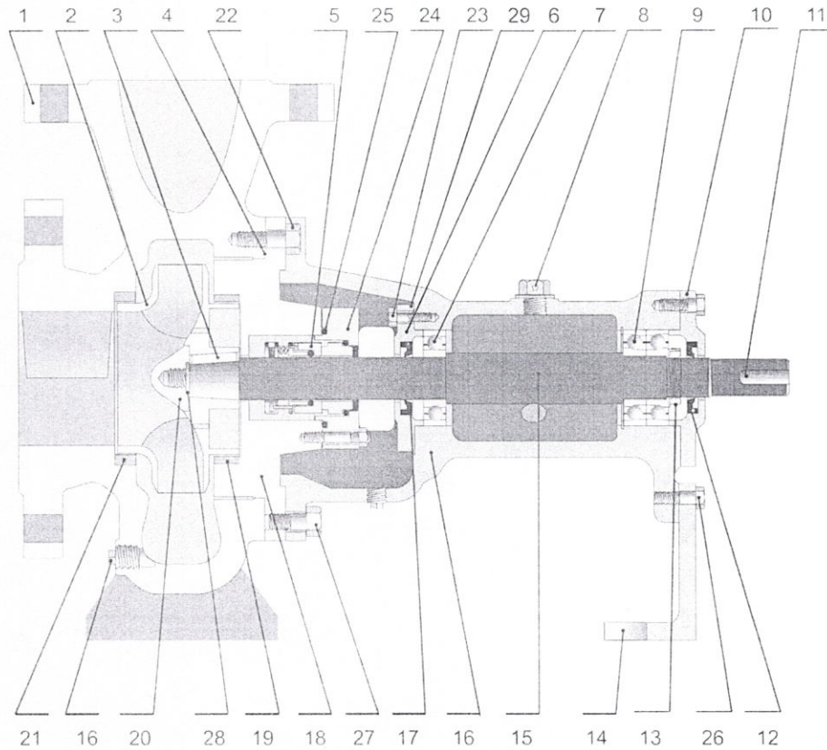
Pump Part List RZ SES SS316 Material
