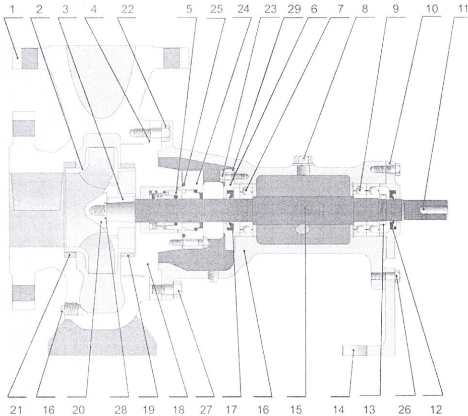
Pump Part List RZ SES SS316 Material
