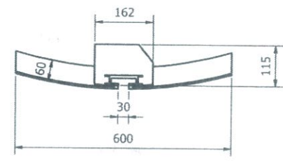
MANHOLE LINER
