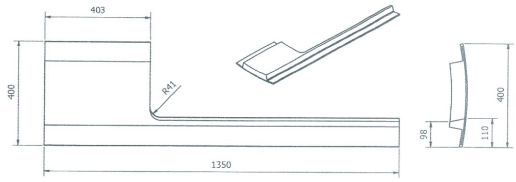
SHELL LINNER SL-C1
