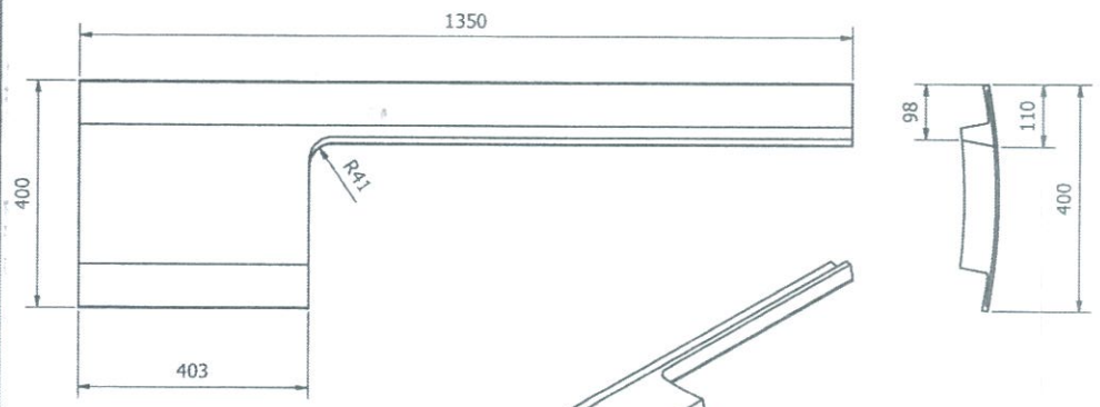
SHELL LINNER SL-C2
