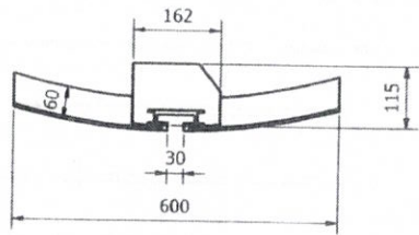
MANHOLE LINER
