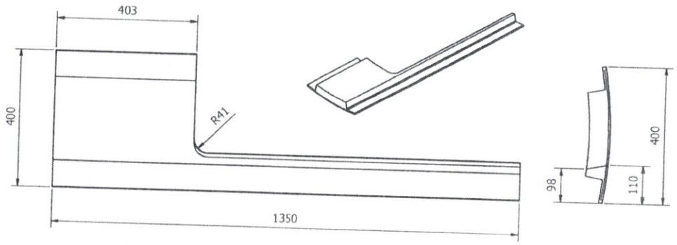
SHELL LINNER SL-C1
